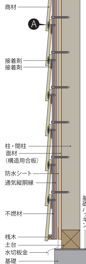
●システム断面図
