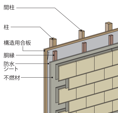
●システム構成図
